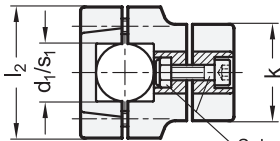
Soket başlı vida / Altıgen somun
