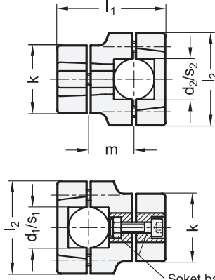
Vida konumları z
